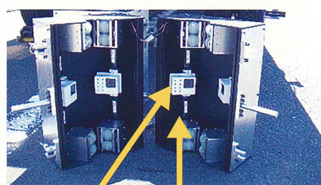
吊橋ハンガーロープの計測例
